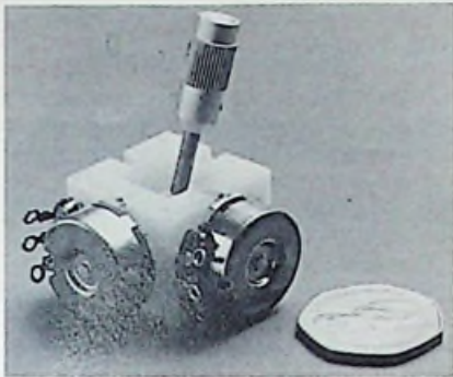
Bild 3. Steuerknüppel-(Joystick-)Potentiometer der A.B. Electronic Components Ltd. zur gleichzeitigen unabhängigen Steuerung zweier Elektronikschaltkreise
