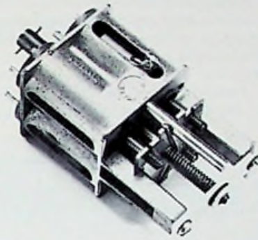
Bild 5. Miniatur-Mittel- und -Langwellen-Tuner von Wingrove & Rogers Ltd.
