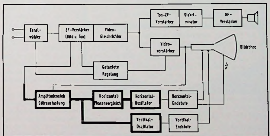
Bild 34. Bei der Fehlererscheinung „Bildschirm hell“ können diese stark umrandeten Stufen defekt sein (Philips)
