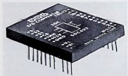
S/D-Konverter SDC-632 der ILC Data Device Corporation
