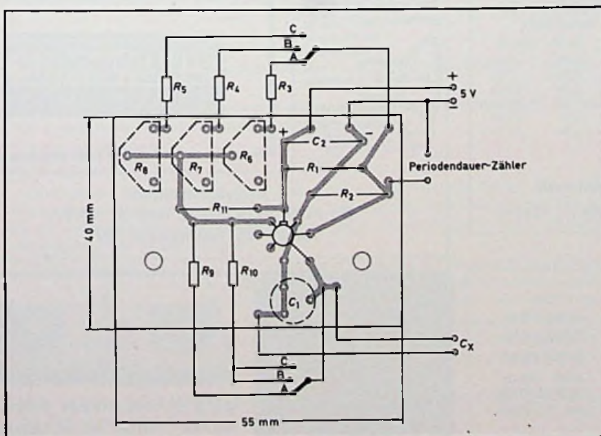
Bild 3. Kapazitätsarme Verbindungen durch Montieren der Platine auf den Bereichsumschalter
