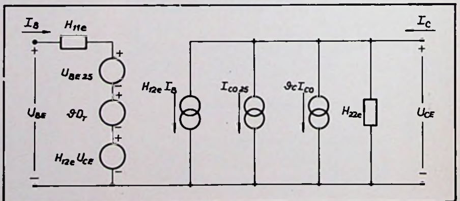
Bild 3. Vollständiges Ersatzschaltbild eines Transistors in Hybridform unter Berücksichtigung des Temperaturverhaltens bei der Emitter-Basis-Schaltung
